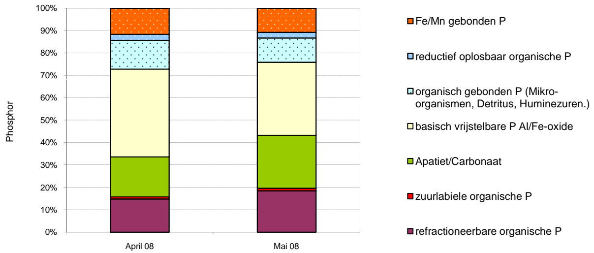
P-gebonden vorm in het sediment van Het Groenen Eiland
